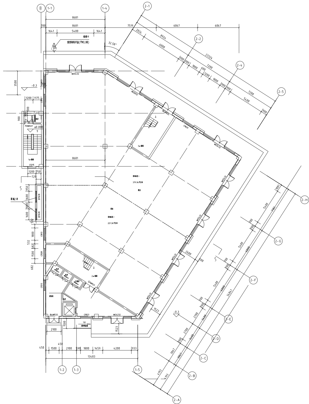
调整前一层平面图
