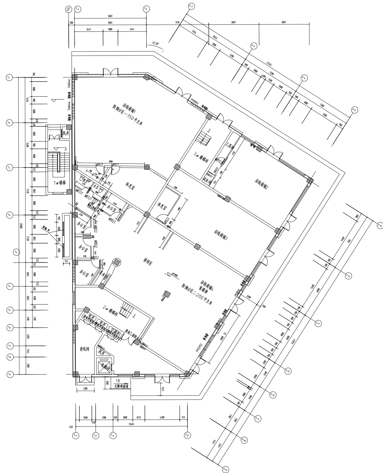
调整后一层平面图
