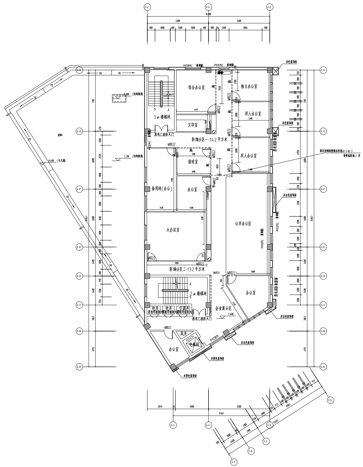
调整后三层平面图
