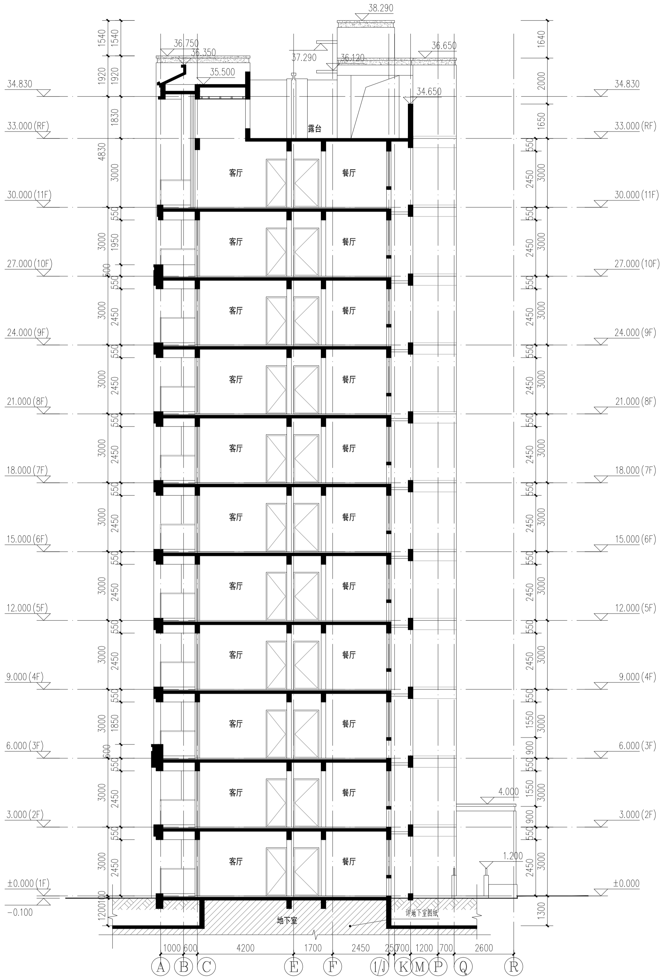
9、12、13#楼 2-2剖面图 1:100
