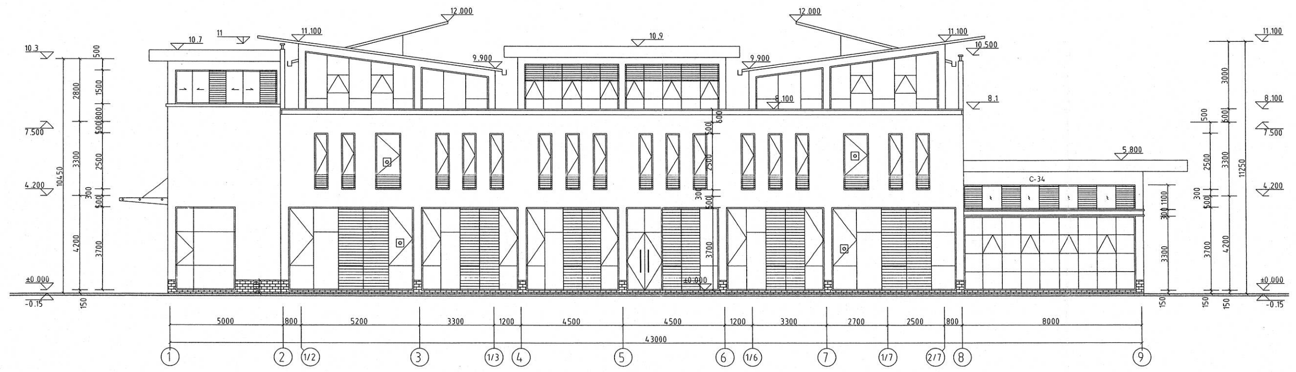
1-9立面图 1:120
